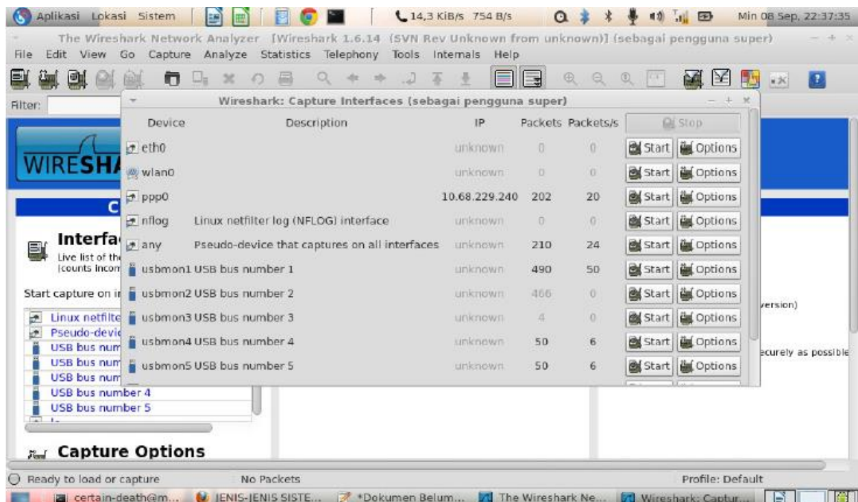
Gambar 3 Memilih interface
